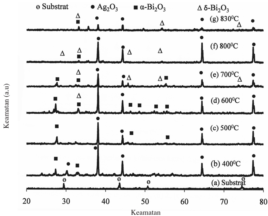
RAJAH 5. Pembelaan sinar-X pada (a) substrat keluli kalis karat dan pada komposit katod \text{Ag}_2\text{O}_3\text{-Bi}_2\text{O}_3 di atas substrat keluli kalis karat dengan empat kali pengulangan salutan dan dirawat pada suhu (b) 400^\circ\text{C} , (c) 500^\circ\text{C} , (d) 600^\circ\text{C} , (e) 700^\circ\text{C} , (f) 800^\circ\text{C} dan (g) 830^\circ\text{C}
